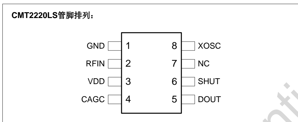
图 1. CMT2220LS 管脚排列图
